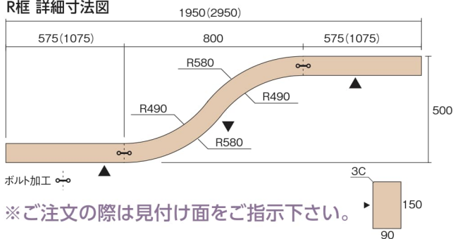
R框 詳細寸法図
