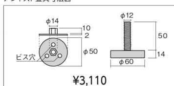
アジャスター金具寸法図
