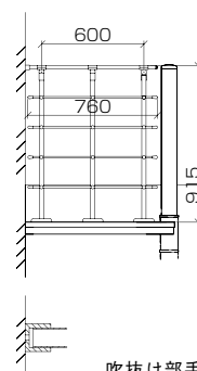
吹抜け部手摺壁納まり
