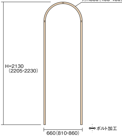
Rアーチ枠 詳細寸法図
