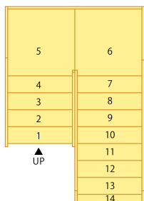
910モジュール【側板納め】仕様明細 ※( )は廻り部巾木納め仕様
