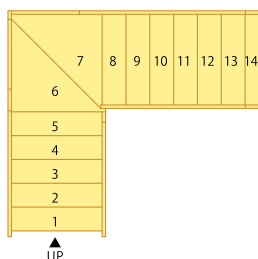
910モジュール【側板納め】仕様明细 ※( )は廻り部巾木納め仕様
