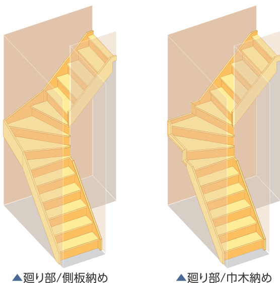
▲廻り部/側板納め
