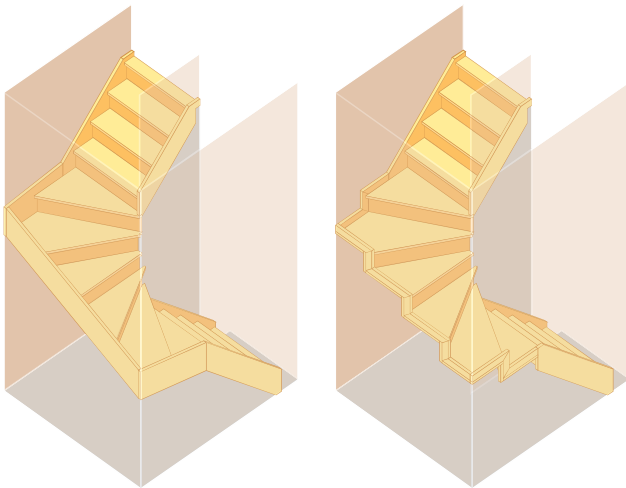
▲廻り部/側板納め
