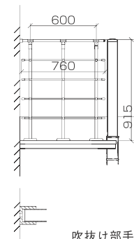
吹抜け部手摺壁納まり
