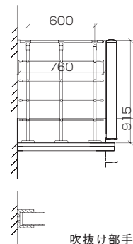
吹抜け部手摺壁納まり
