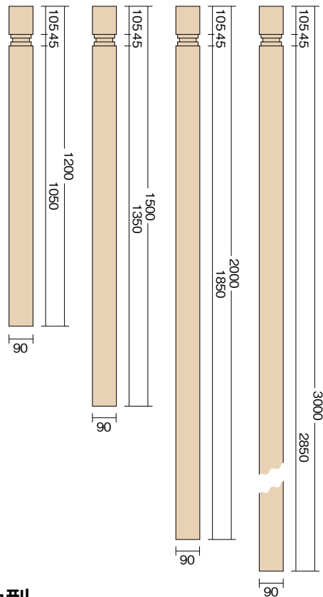
90mm角型
