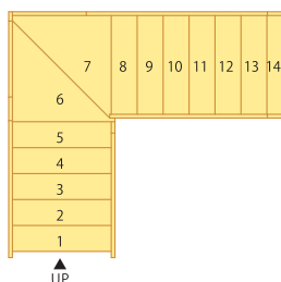
910モジュール【側板納め】仕様詳細 ※( )は廻り部巾木納め仕様
