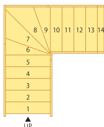
910モジュール【側板納め】仕様詳細 ※( )は廻り部巾木納め仕様
